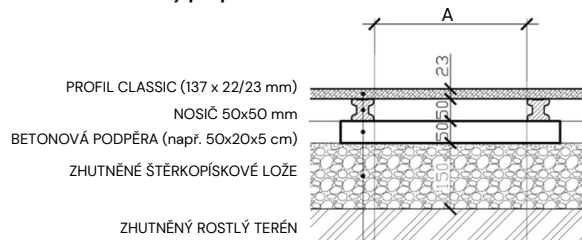
Obr. 1 Skladba terasy při použití nosičů GRANDECK® 50x50 mm
