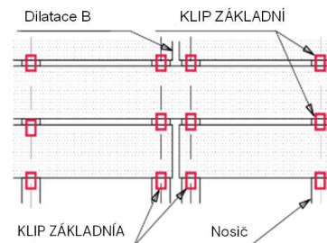
Obr. 5 Napojování terasových prken pomocí ZÁKLADNÍHO KLIPU
