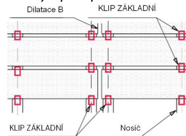
Obr. 5 Napojování terasových prken pomocí ZÁKLADNÍHO KLIPU
